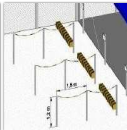
Estacionamento de veículos utilizando poste metálico e batente de concreto.
