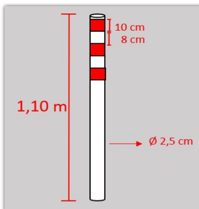
Especificação do poste em PVC.
